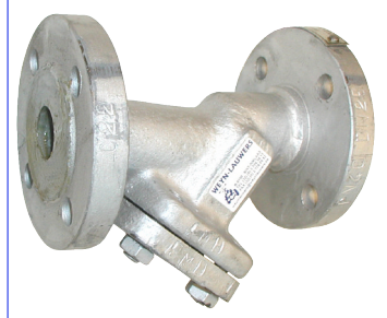
stalen ANSI Y-filters inox zeef huis : ASTM A216"WCB temp. : -20°C +400°C fig 808 : ansi 150 lbs / 2" - 12" fig 809 : ansi 300 lbs / 2" - 12"
