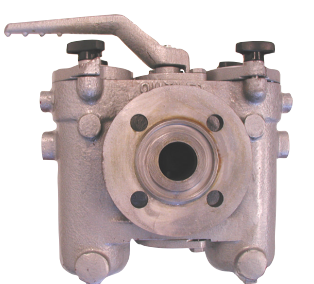
wisselfilter PN16 huis in gietijzer zeven in inox fig 834 : DN25 - DN150 flenzen volgens PN16
