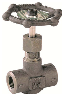
naaldventiel staal PN210 A105/F6 smeedstaal 1/4" - 1" ANSI 3000 lbs grafiet spindelafdichting / naald : inox 316 temp. : -20°C/+250°C fig 526 bsp draadaansluiting fig 527 npt draadaansluiting fig 528 SW laseinden
