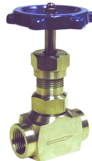
fig 521 naaldventiel staal PN210 1/4" - 1" bsp ANSI 3000 lbs huis : staal A105 teflon spindelafdichting naald : inox 316 temp. : -20°C/+250°C
