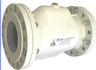
fig 686 mofafsluiter aluminium DN 40 - DN 200 huis : aluminium mof : natuurrubber flenzen volgens PN10 max. werkdruk 6 bar stuurdruk : = werkdruk + 2 bar temp. : max. +80°C voedingsgeschikte rubber op aanvraag
