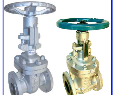
fig 375 staal / schuifafsluiter 150 lbs huis staal ASTM A216/WCB TRIM 8 flenzen volgen ANSI 150 LBS 1/2" - 12" temp. : -29°C/+425°C fig 376 : 300 lbs
