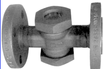
fig 886 stalen kijkglas PN40 geflensd DN15 - DN40 huis : staal A105 temp. : -10°C +300°C max. druk 40 bar voor dn15 en dn20 max. druk 20 bar voor dn25, dn32 en dn40 dubbel borosilicaat glas
