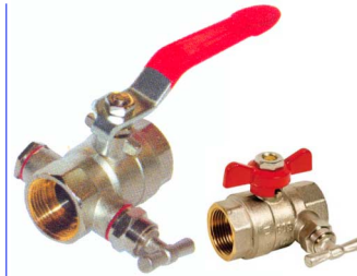
messing volle doorlaat met aflaat fig 97 : FF 1/2" - 2" bsp fig 97BF : FF - vleugelhendel 1/2" - 1" FF
