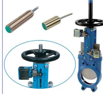
eindschakelaars mechanisch met rolstiftbediening of met naderingsschakelaars PNP NO 3-draads
