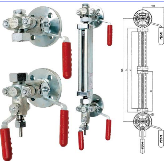
boven- en onderkraan voor niveuaanduiding huis en flenzen : staal A105 flenzen PN40 fig 873 : DN 15 - DN 20 - DN 25 voorzien van aftaalkraan aansluiting op buisjes diam. 16 mm
