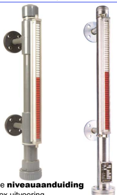
fig 891 inox niveuaanduiding (zonder glas) 3/8" - 1/2" - 1" bsp inox 316 naaldventiel en bocht max. druk 16 bar / temp. : -50°C +200°C viton en teflon afdichtingen fig 890 messing niveuaanduiding 1/4" - 3/8" - 1/2" - 3/4" bsp max. 6 bar/80°C
